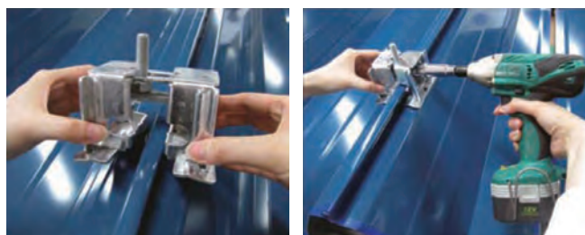
写真5 折板へのPVパネル固定用金具 7)
