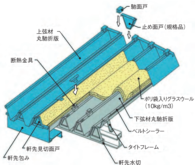
図2 断熱2重折板
